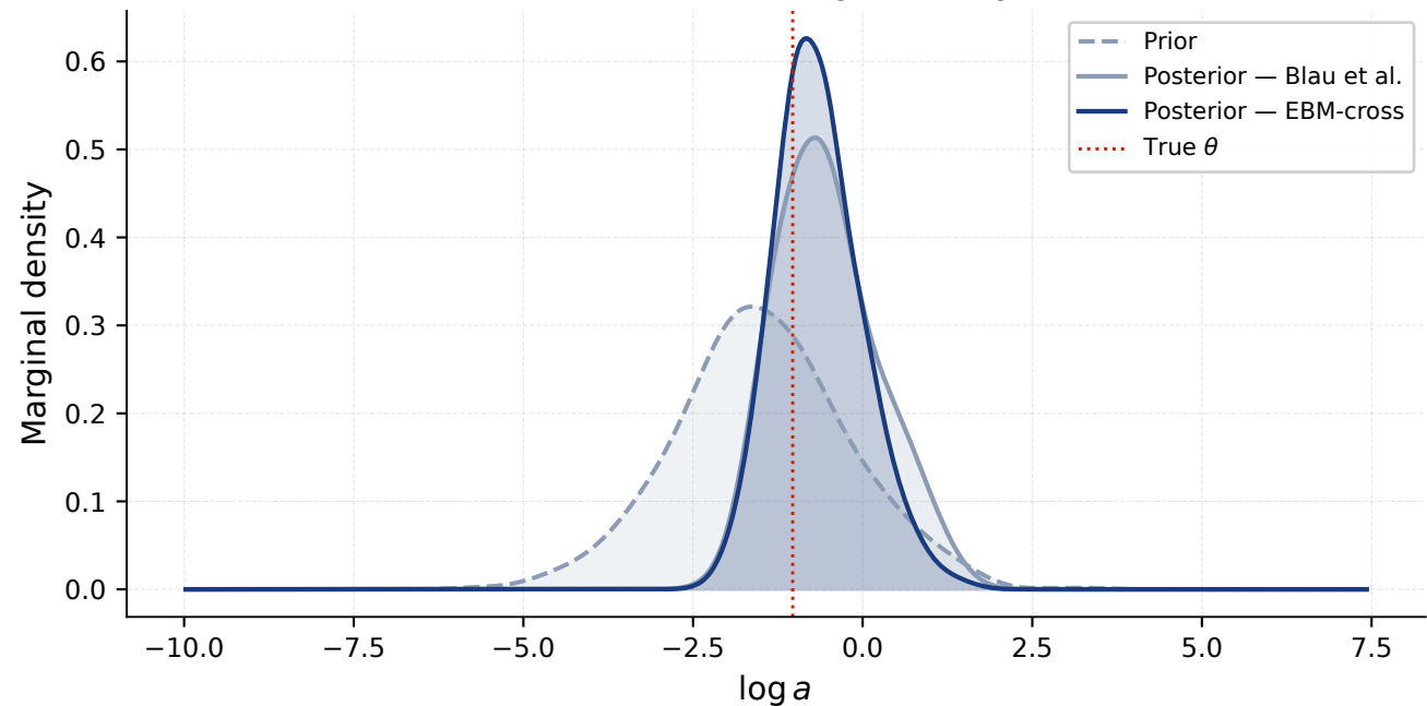
Prior vs Posterior marginals — \log a
