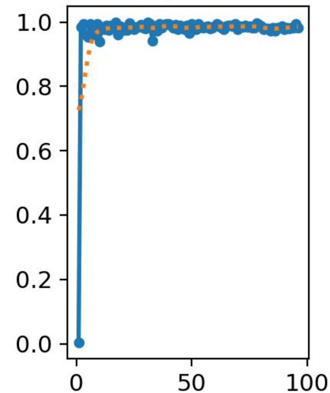
metrics/precision(B)
