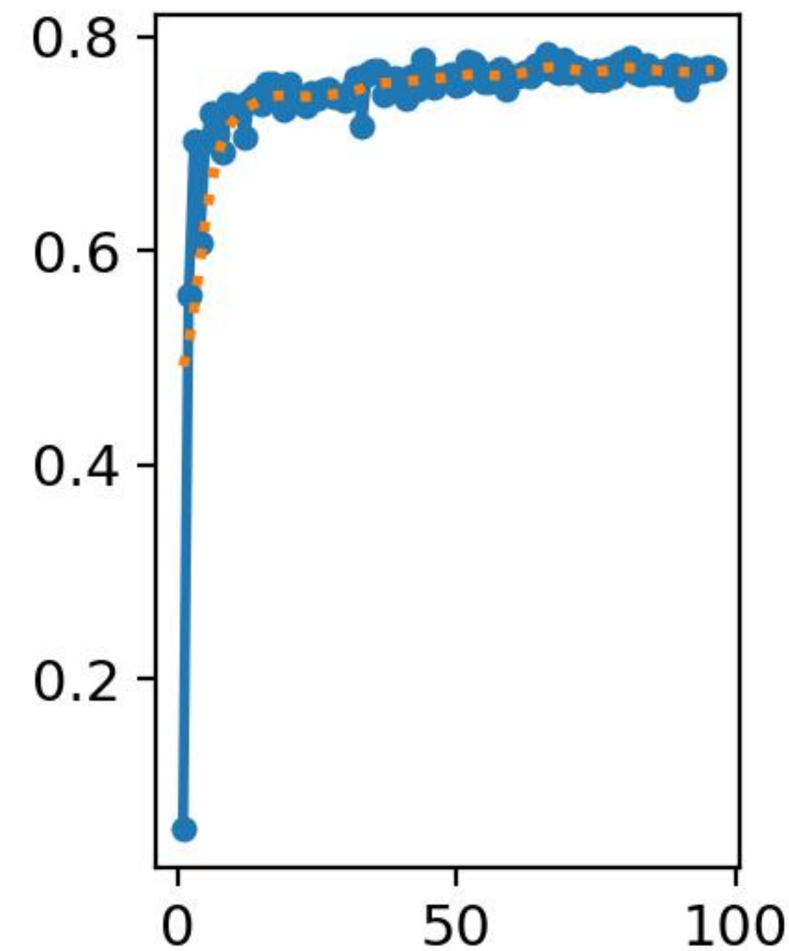
metrics/mAP50-95(B)
