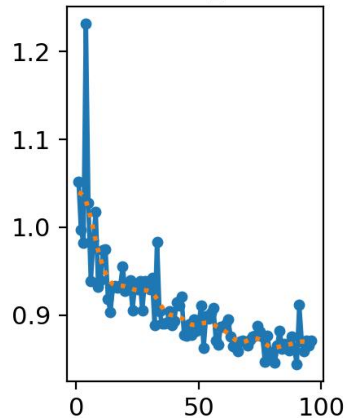
val/box_loss
