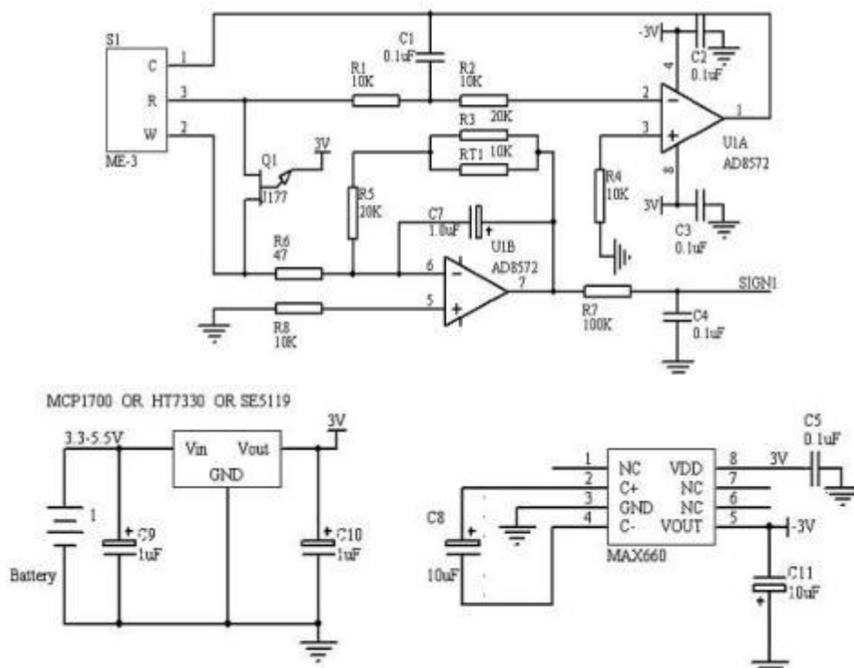
图 2： ME3-SO 2 测试电路
