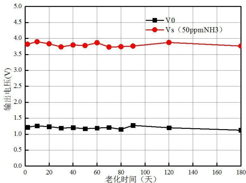
图 7 长期稳定特性曲线
