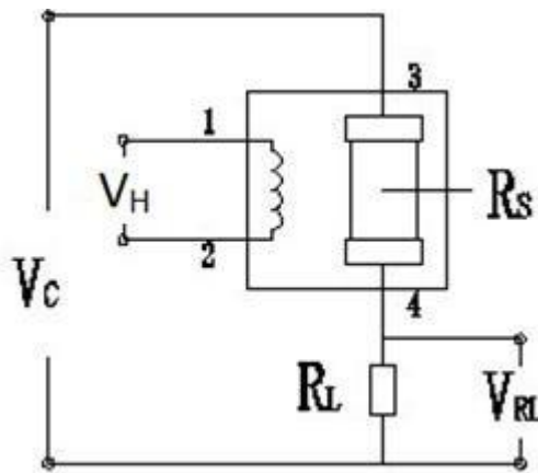
图 2 MP-702 测试电路
