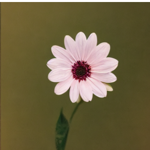
Diffusion-DPO
