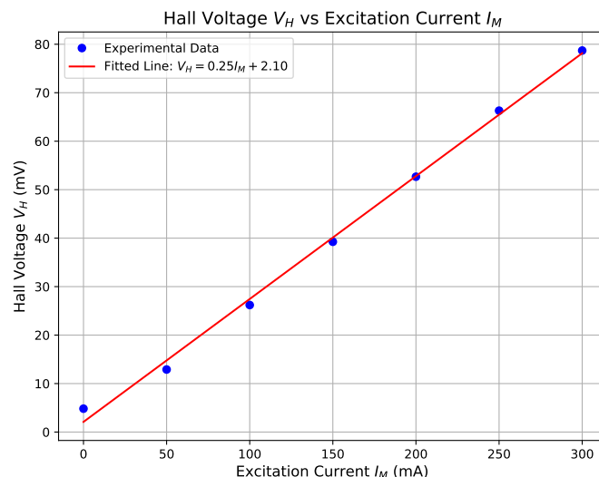
图 4: 霍尔电压 V_H 与励磁电流 I_M 关系曲线
