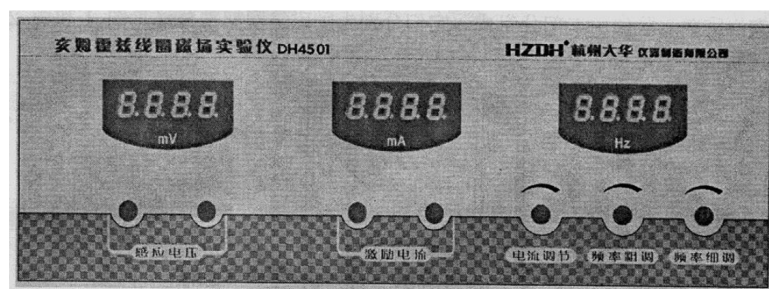
图 10：DH4501 亥姆霍兹线圈磁感应强度测量仪面板
