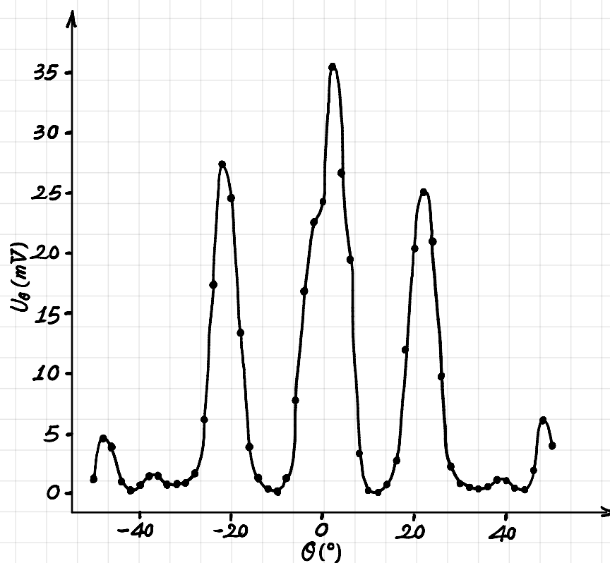
图3. 双缝干涉实验
