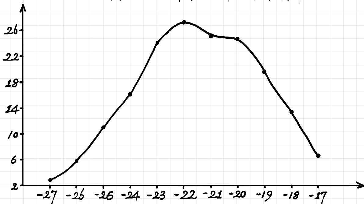
图 4-1 双缝干涉一级极大扫描结果
