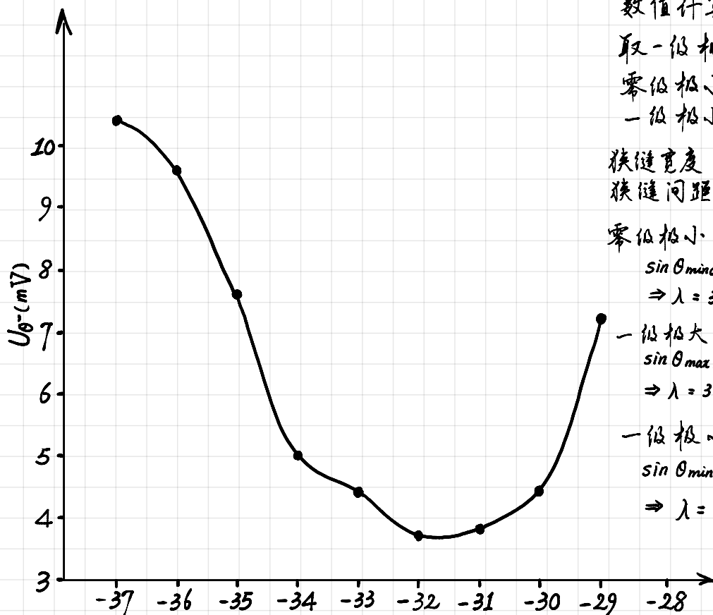
图6-1 双缝干涉一级极小扫描结果
