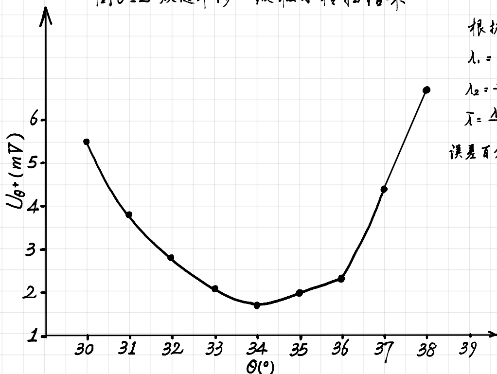
图6-2 双缝干涉一级极小扫描结果
