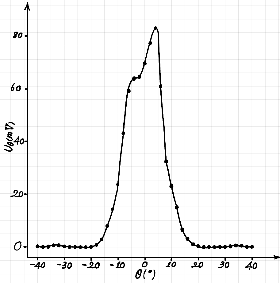
图1: 单缝衍射实验数据
