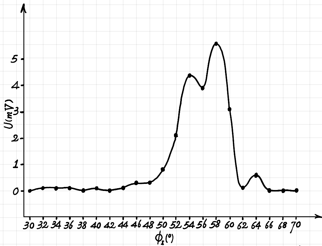
圖 11 (100) 晶面在极大值附近的精扫
