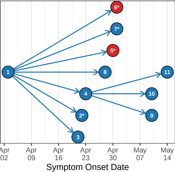
Tree 4 – 0.14% of posterior
