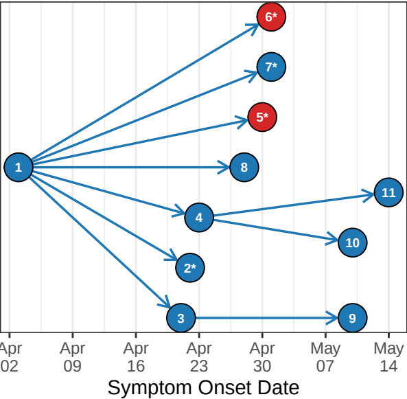
Tree 3 – 0.15% of posterior
