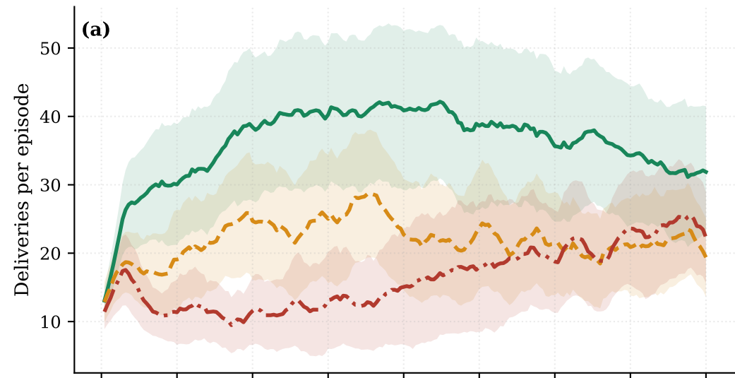
IPPO
