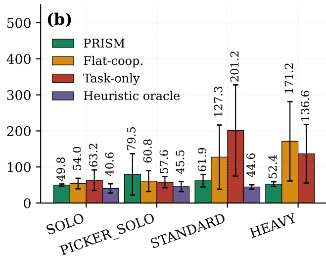
MAPPO
