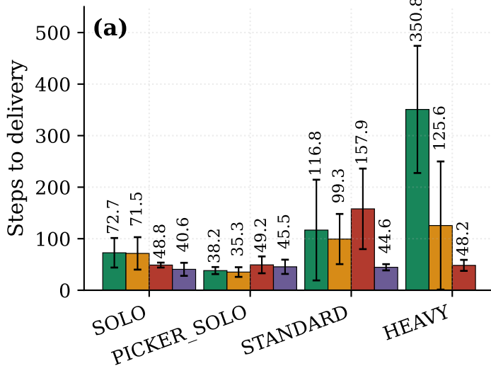
IPPO
