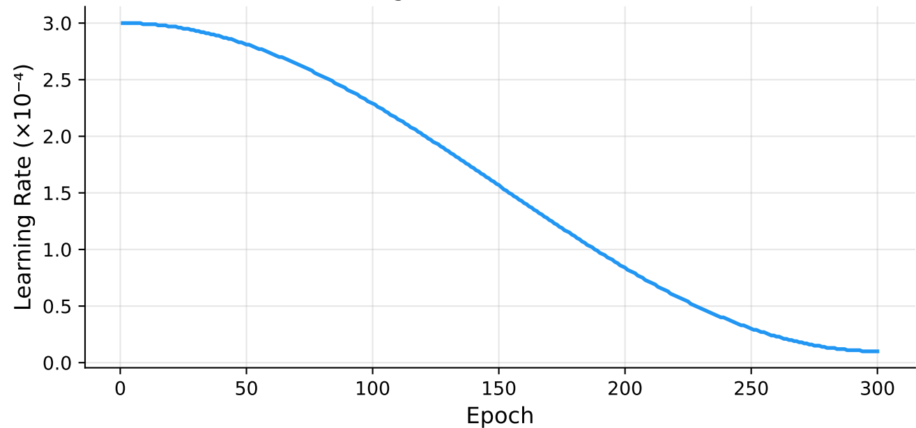
CosineAnnealingLR Schedule ( 3 \times 10^{-4} \rightarrow 1 \times 10^{-5} )
