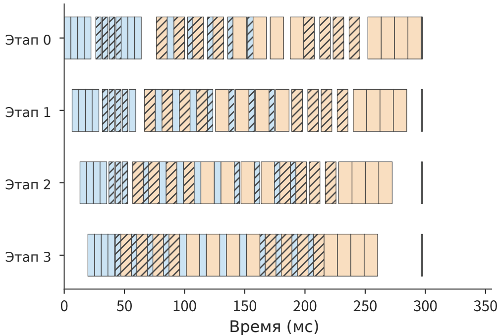
Чередующийся 1F1B ( v=2 ): 298 мс
