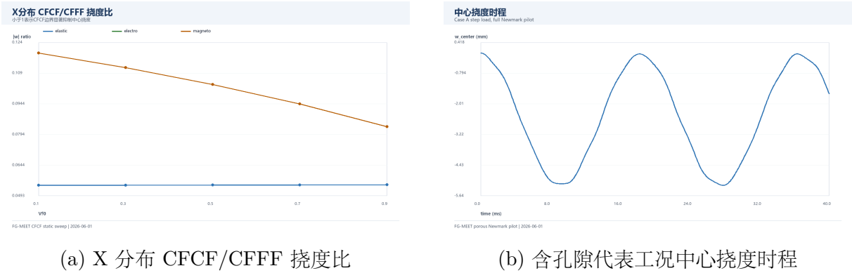
图 7: 新增边界条件和含孔隙动力结果
