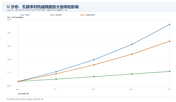
(a) U 分布挠度倍率
