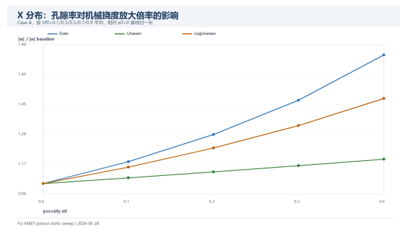
(b) X 分布挠度倍率
