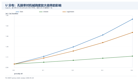
(a) U 分布挠度倍率
