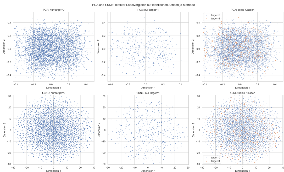
Abbildung 8: PCA- und t-SNE-Projektionen nach Targetklasse. Die Punktwolken überlappen deutlich. Die zweidimensionale Darstellung liefert deshalb keine klare Targettrennung.
