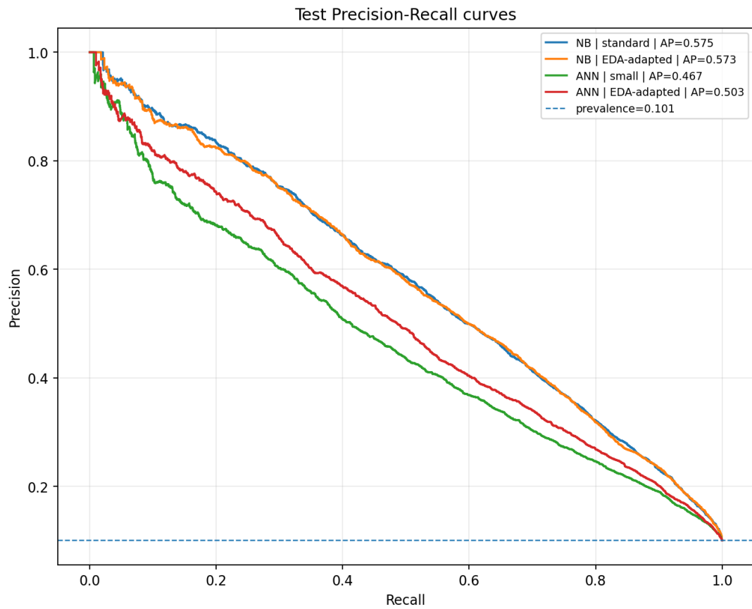
Abbildung 13: Precision-Recall-Kurven auf dem internen Testsplit. Bei einer Positivrate von 0,101 erreichen die NB-Varianten mit AP 0,575 und 0,573 die besten Werte.
