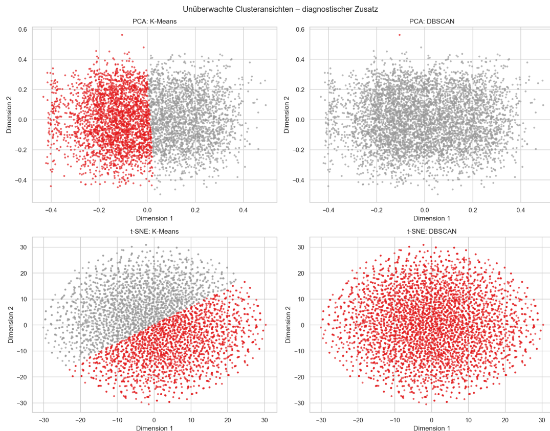
Abbildung 9: K-Means- und DBSCAN-Ergebnisse in PCA- und t-SNE-Räumen. ARI und NMI liegen ungefähr zwischen -0,0007 und 0,0008 . Die Cluster stimmen damit praktisch nicht mit dem Target überein.
