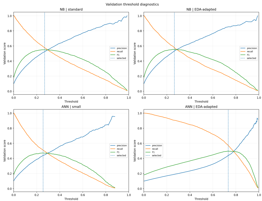
Abbildung 14: Threshold-Diagnostik auf den Validierungsdaten. Die gestrichelte Linie markiert je Modell die gewählte Schwelle nahe dem höchsten F1-Wert und zeigt den zugehörigen Precision-Recall-Kompromiss.
