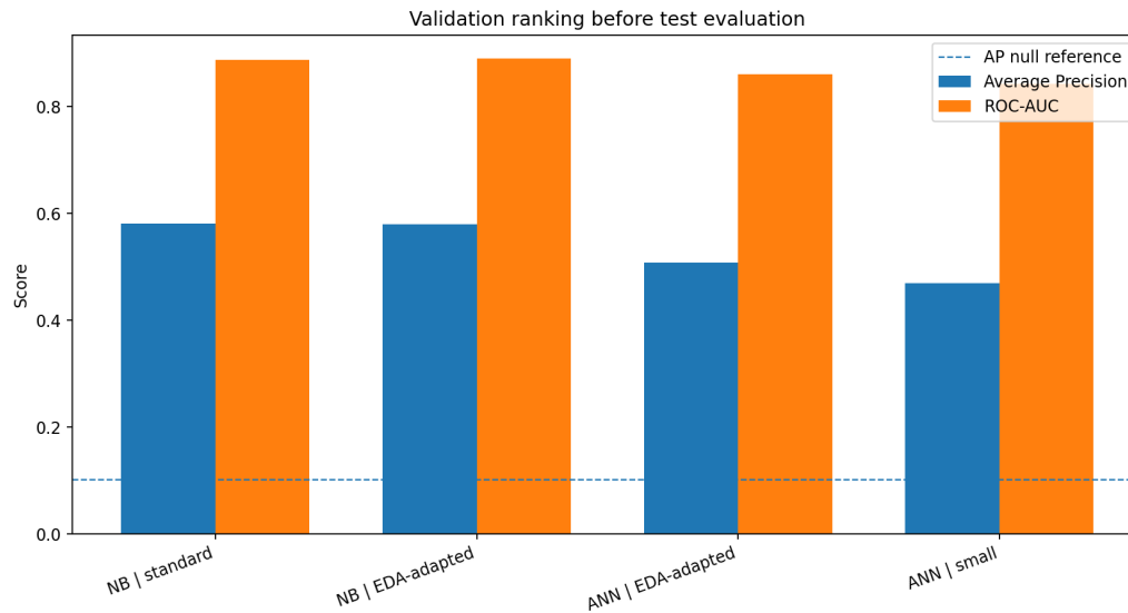
Abbildung 10: Validation-Ranking der vier Modelle. Das einfache Standard-GaussianNB liegt nach der vorab festgelegten AP vorn; weder Quantiltransformation noch höhere ANN-Komplexität rechtfertigen einen Wechsel.
