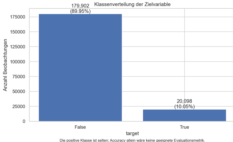
Abbildung 5: Klassenverteilung des Targets. Eine triviale Negativvorhersage wäre bereits etwa 90 % korrekt; deshalb werden PR/AP, Balanced Accuracy und klassenbezogene Fehler benötigt.
