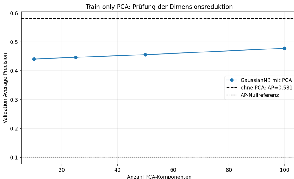
Abbildung 17: Train-only PCA-Vergleich. Keine der geprüften Kompressionen erreicht die Validation-AP des Modells ohne PCA; der Informationsverlust überwiegt den möglichen Regularisierungsvorteil.
