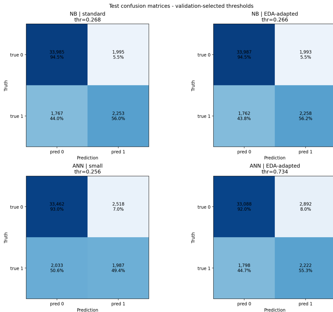
Abbildung 11: Confusion Matrices bei den auf Validation bestimmten Schwellen. Die Matrizen zeigen die Anzahl der False Positives und False Negatives und machen sichtbar, dass ein besseres Ranking nicht automatisch denselben Betriebspunkt bedeutet.
