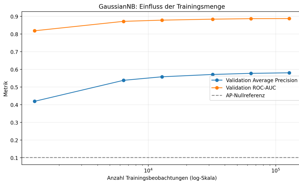
Abbildung 16: Learning Curve des Standard-GaussianNB. Kleine Vorläufe liefern bereits ein sinnvolles Signal; mehr Trainingsdaten verbessern AP weiter, der Zugewinn flacht jedoch sichtbar ab.
