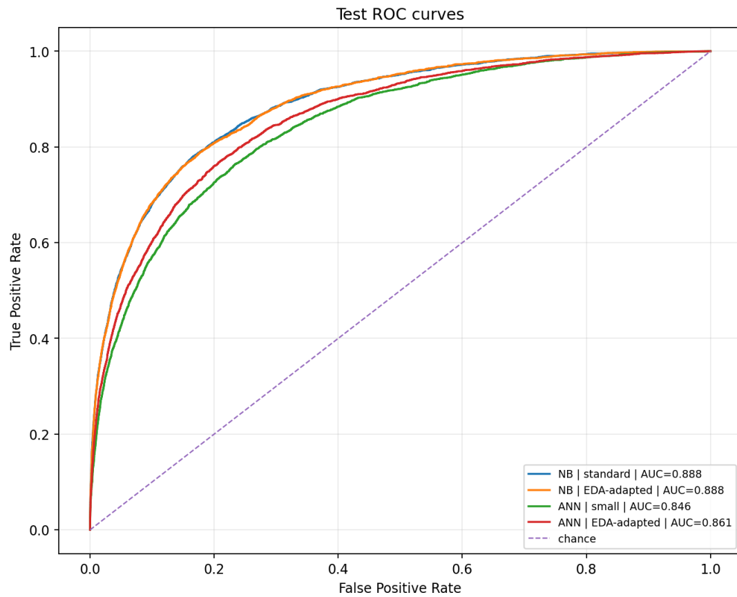
Abbildung 12: ROC-Kurven auf dem internen Testsplitt. Beide NB-Varianten erreichen eine ROC-AUC von rund 0,888 und liegen vor den ANN-Varianten.
