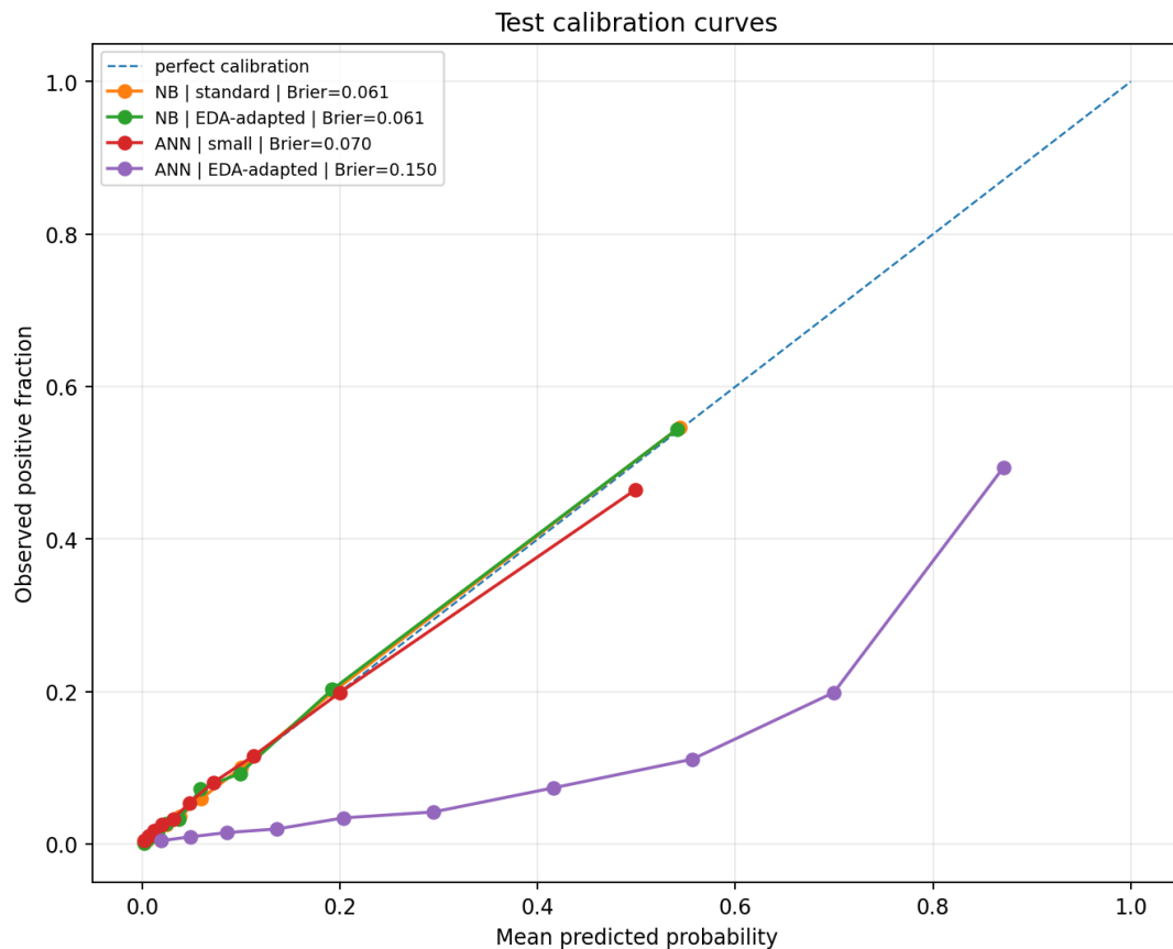
Abbildung 15: Kalibrierungskurven auf dem internen Testsplit. Die NB-Varianten liegen mit einem Brier-Score von rund 0,061 nahe an der Ideallinie. Das EDA-ANN weicht mit 0,1505 deutlich stärker ab.
