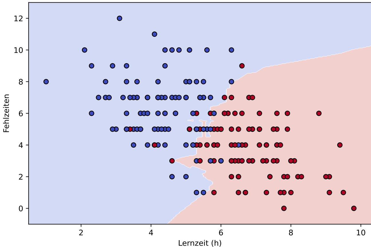
KNN-Entscheidungsgrenze (k=5)
