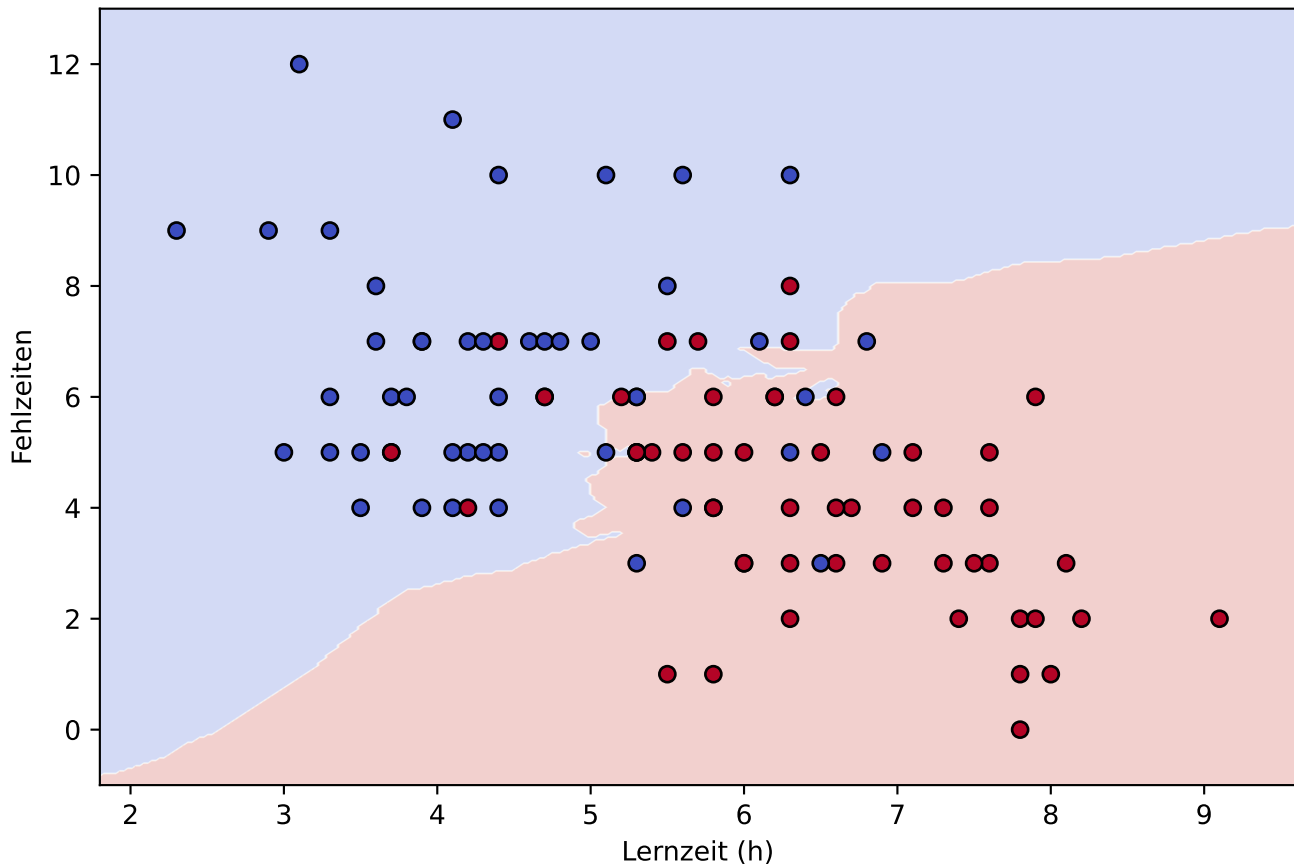
KNN-Entscheidungsgrenze (k=15)
