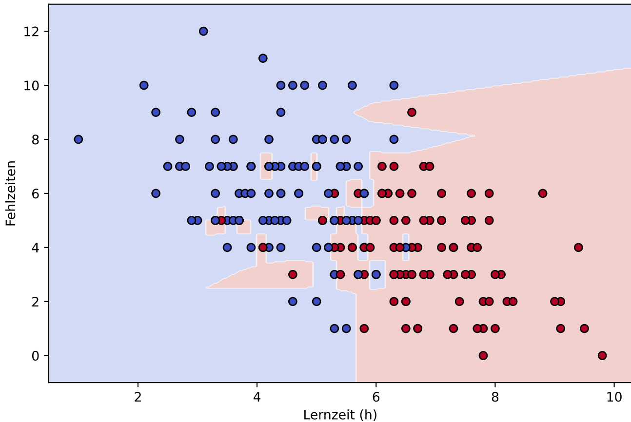
KNN-Entscheidungsgrenze (k=1)
