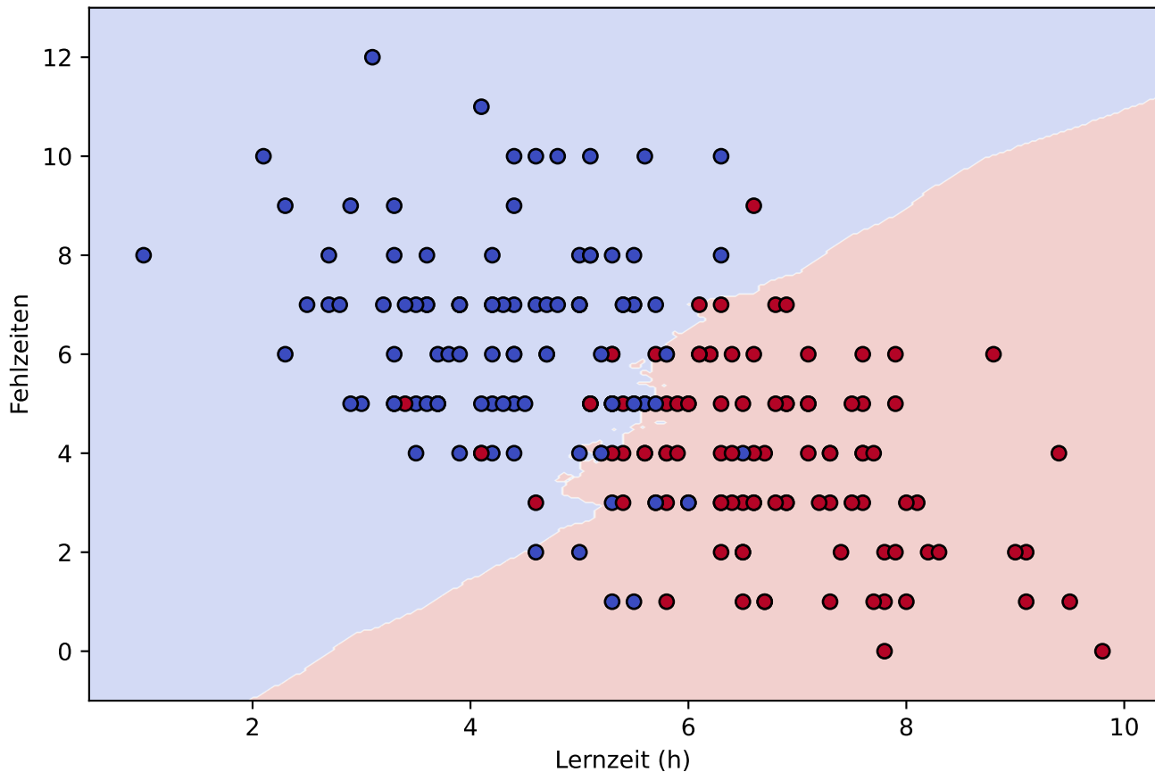
KNN-Entscheidungsgrenze (k=15)
