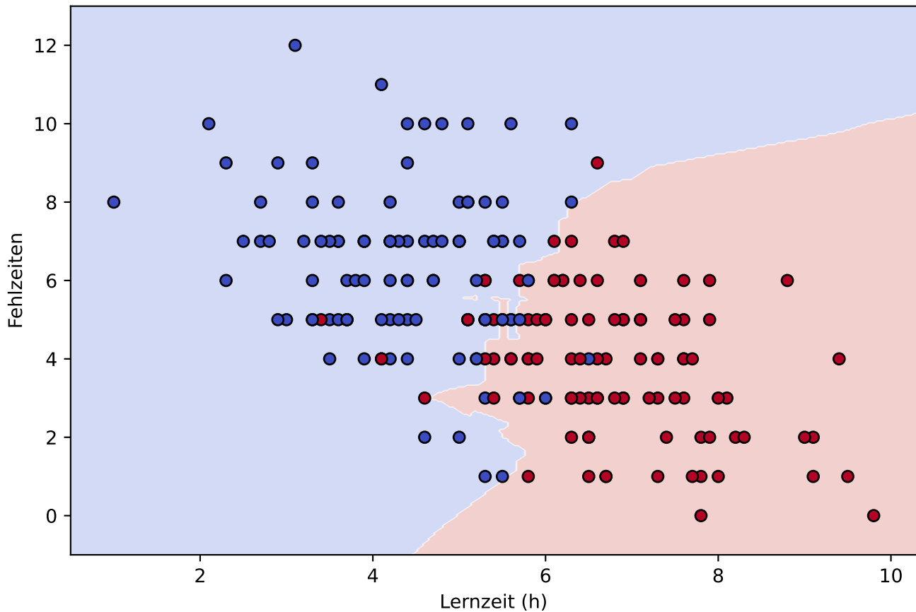
KNN-Entscheidungsgrenze (k=5)
