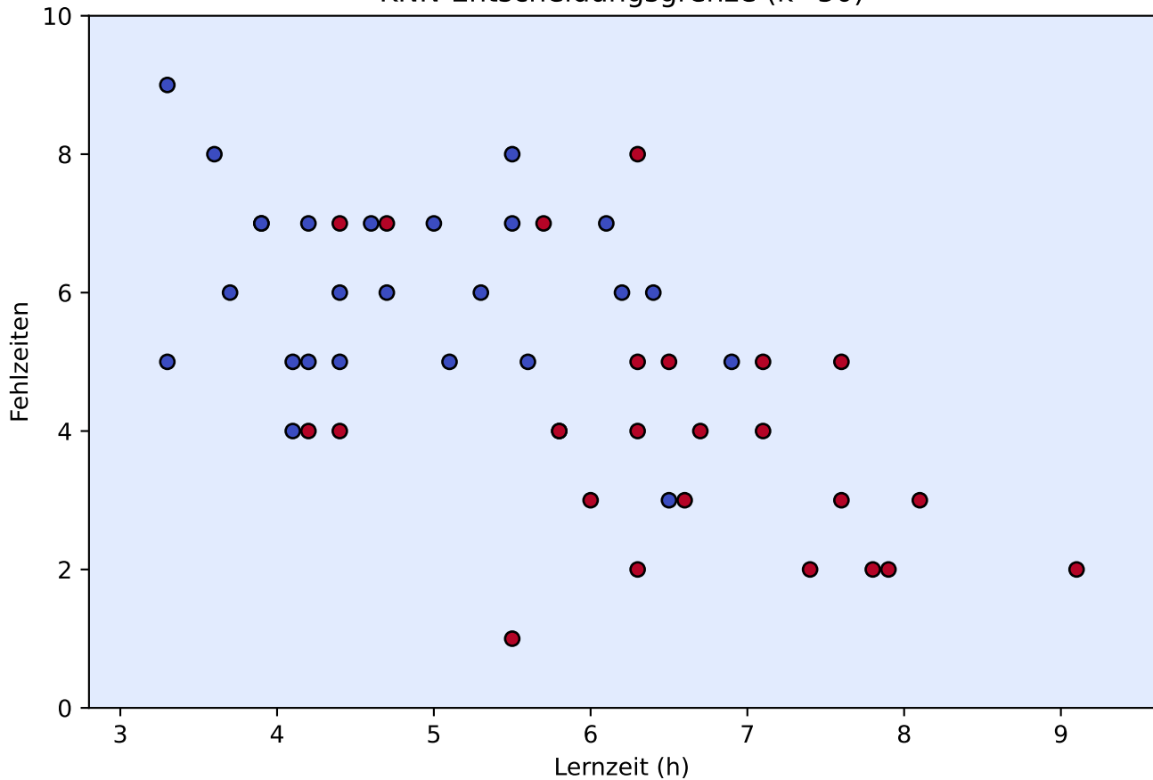
KNN-Entscheidungsgrenze (k=50)
