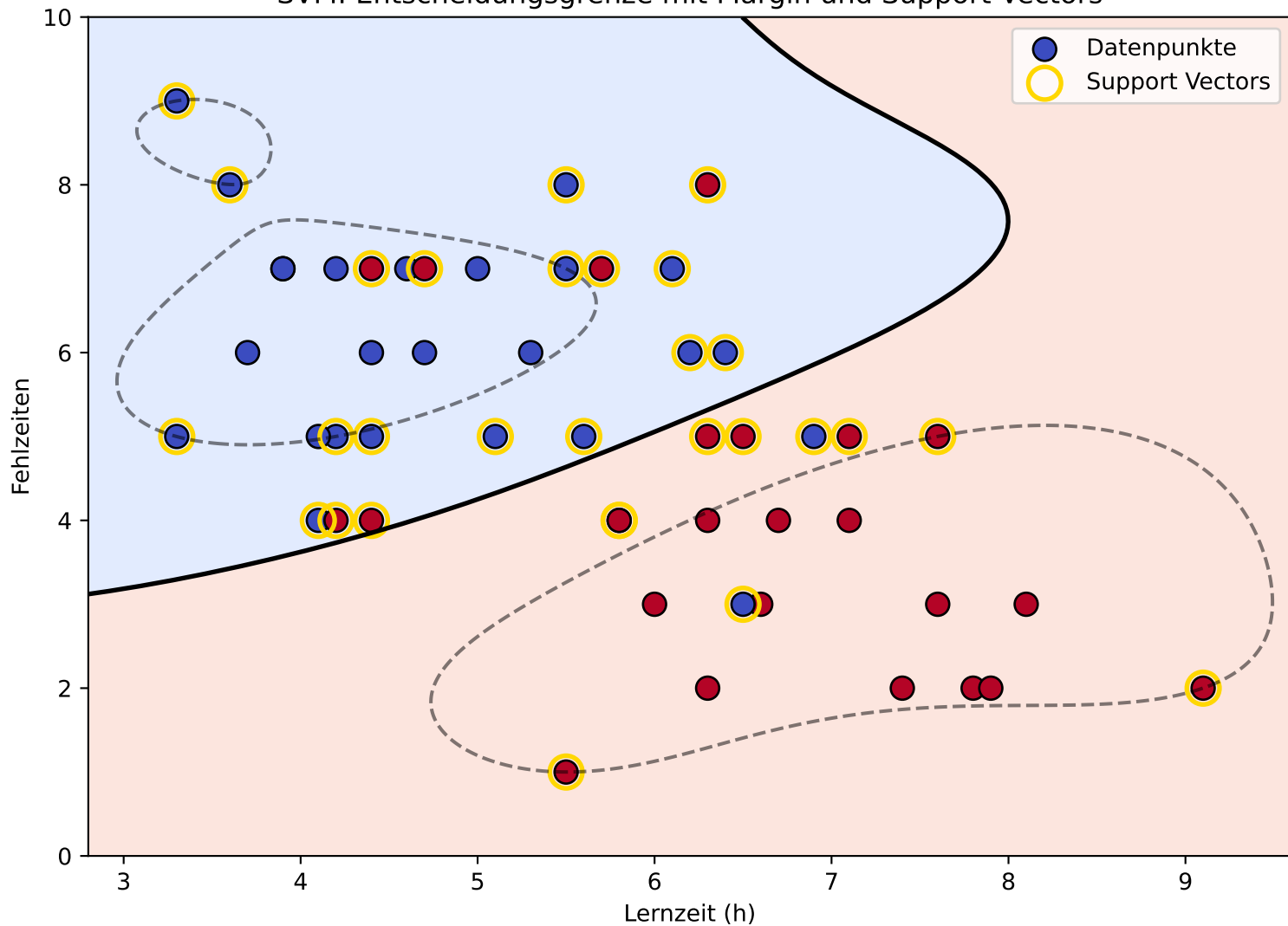
SVM: Entscheidungsgrenze mit Margin und Support Vectors
