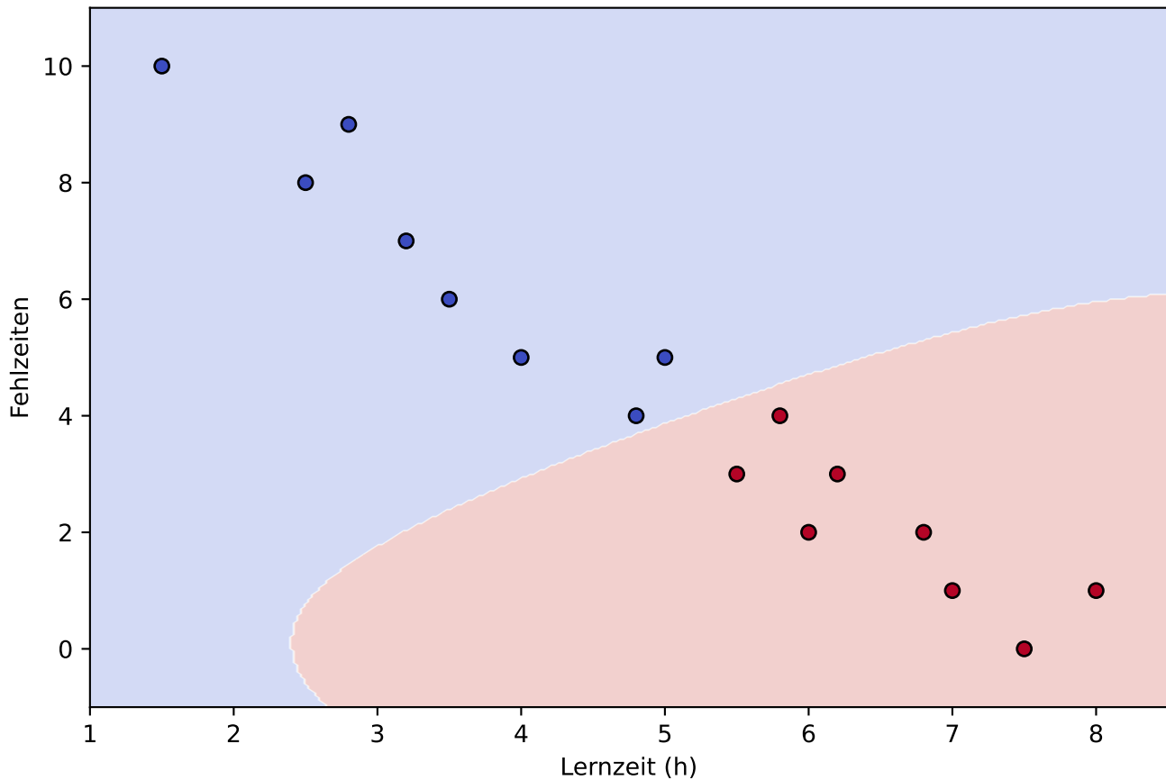
SVM-Entscheidungsgrenze
