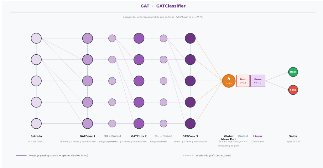
Figura 2.3: Arquitetura da GAT utilizada neste trabalho: três camadas GATConv com atenção softmax multi-cabeça (camadas 1 e 2: 4 cabeças, concat=False; camada 3: 1 cabeça), seguidas de Global Mean Pool, Dropout (0,5) e classificador linear (64→2).
