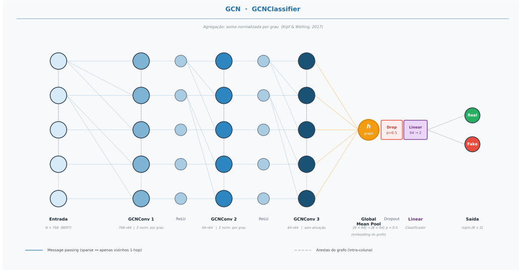
Figura 2.2: Arquitetura da GCN utilizada neste trabalho: três camadas GCNConv ( 768 \rightarrow 64 , 64 \rightarrow 64 , 64 \rightarrow 64 ) com ativação ReLU, seguidas de Global Mean Pool, Dropout (0,5) e classificador linear ( 64 \rightarrow 2 ).
