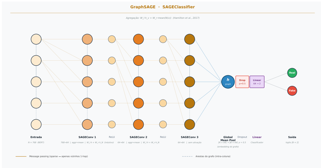
Figura 2.4: Arquitetura da GraphSAGE utilizada neste trabalho: três camadas SAGEConv com agregação por média ( W_l \cdot h + W_r \cdot h_N , indutivo), seguidas de Global Mean Pool, Dropout (0,5) e classificador linear (64→2).
