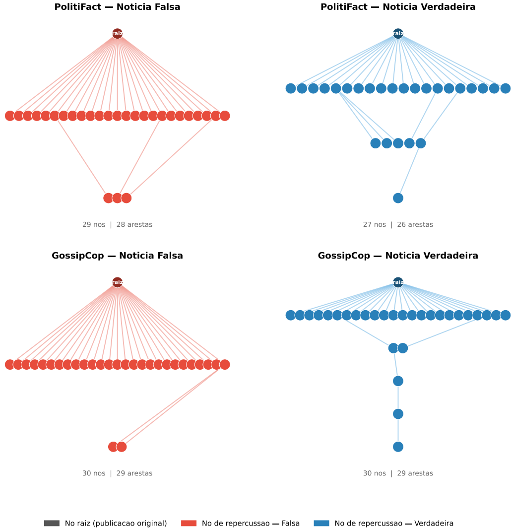
Figura 2.1: Exemplos reais de árvores de propagação extraídos dos conjuntos UPFD PolitiFact (linha superior) e GossipCop (linha inferior). O nó raiz (mais escuro) representa a publicação original; os demais nós representam interações subsequentes (reposts, respostas). Em ambos os datasets, exemplos falsos (vermelho) e verdadeiros (azul) apresentam estruturas superficialmente similares em tamanho — evidenciando que o número de nós isolado não é discriminante, motivação central para o uso de GNNs neste trabalho.
