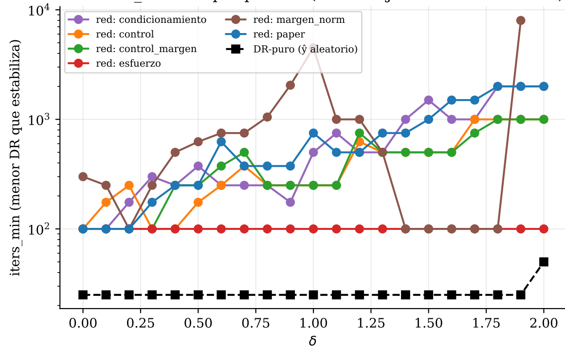
P1 · \text{iters\_min} vs \delta por pérdida (banda roja = CVXPY infactible)
