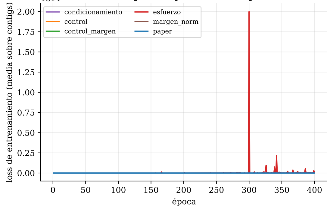
Curvas de pérdida por función de pérdida
