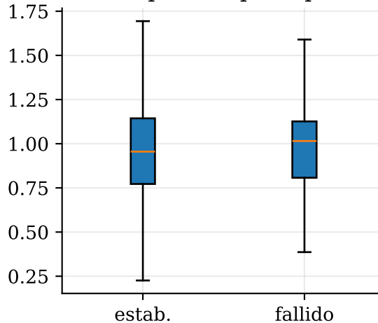
dispersión politopo
