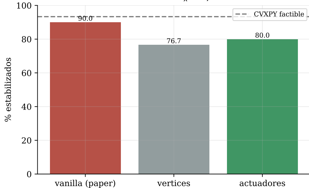
Celda comun n_x = 3, N = 2
