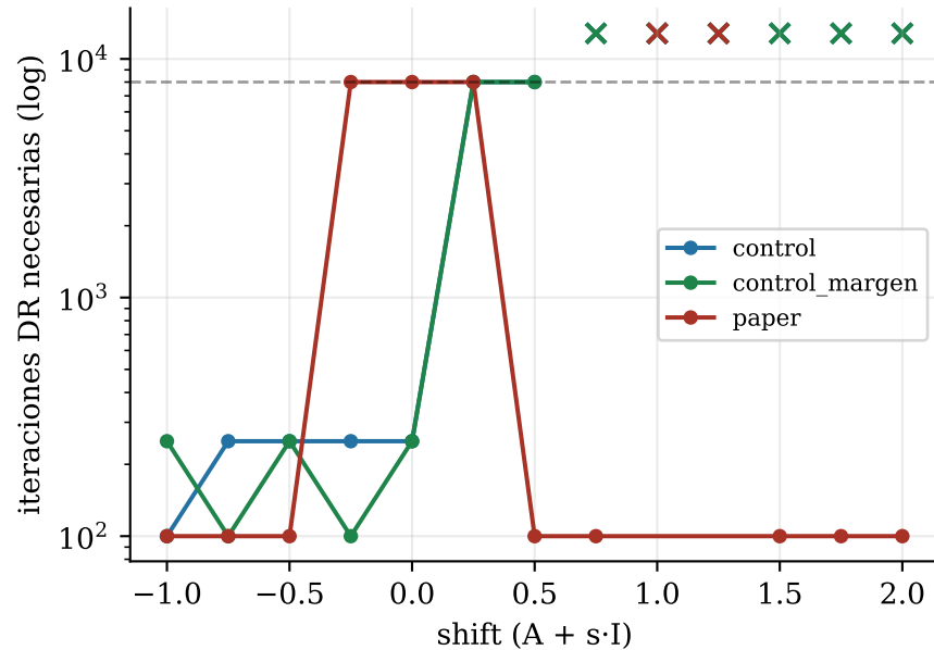
Costo de iteraciones (x = no logrado)
