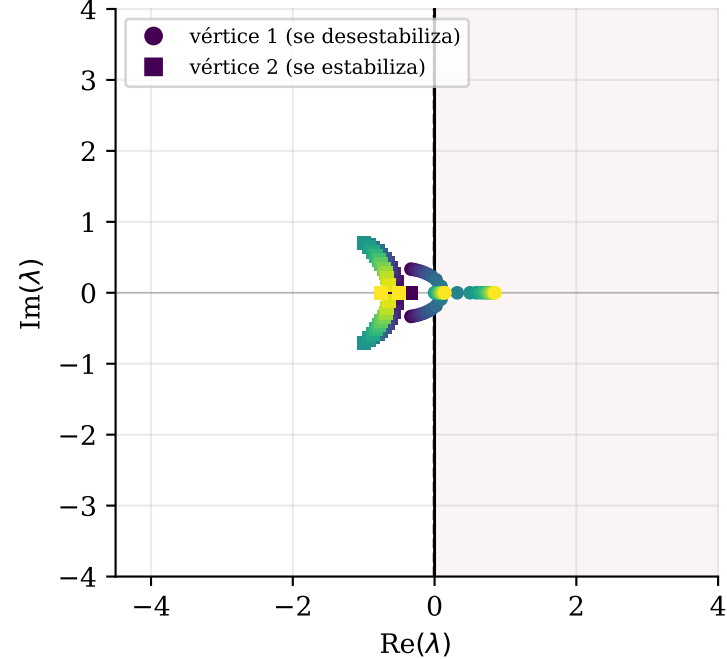
A. Lazo abierto: migración de polos con \delta
