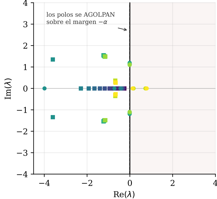
B. Lazo cerrado de la red (`control`)
