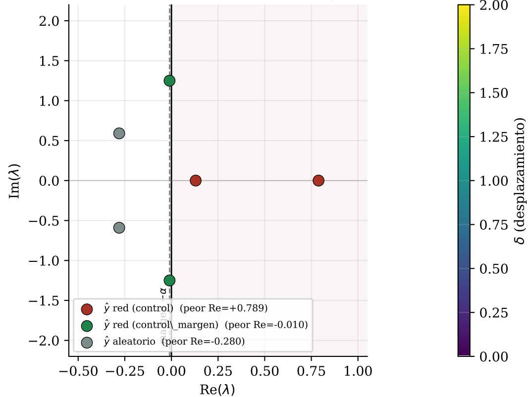
C. \delta = 2 : dónde aterriza cada \hat{y}
