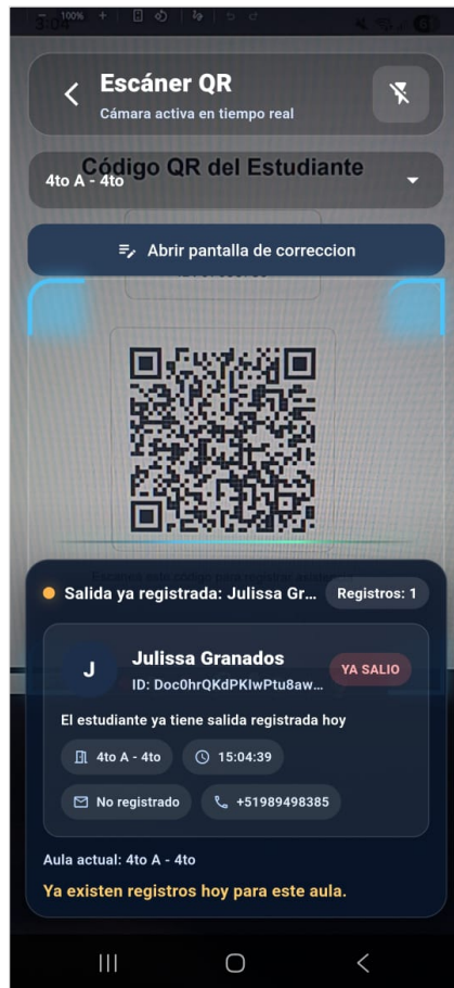
Figura 6. Resultado de un segundo escaneo del mismo alumno: el sistema reconoce el duplicado y muestra el estado correspondiente sin alterar el registro.
