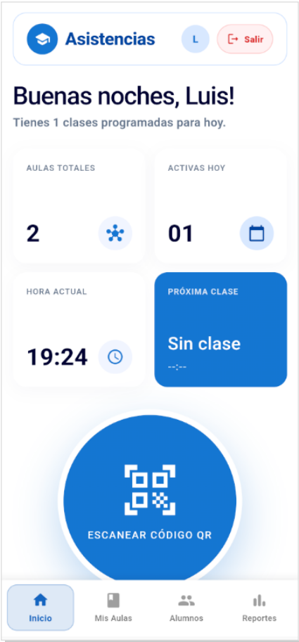
Figura 2. Panel principal del docente. La barra inferior contiene los accesos a Inicio, Mis Aulas, Alumnos y Reportes.
