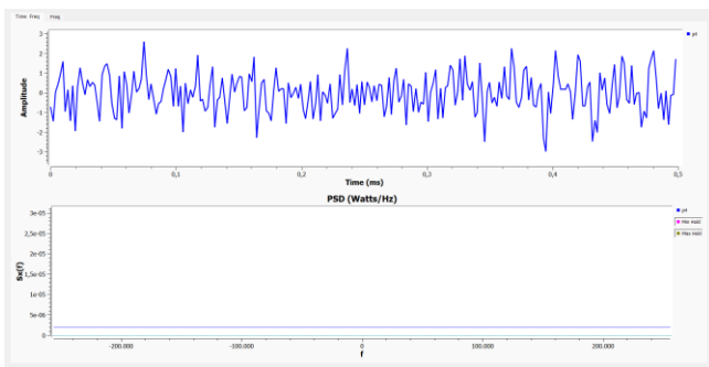
Figura 4. Señal a ruido blanco sps = 16
