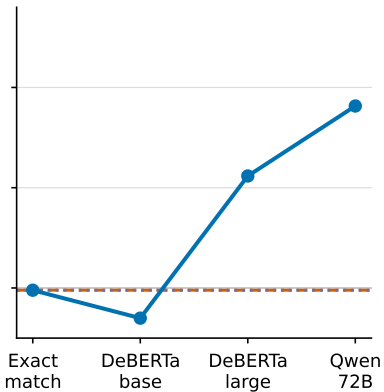
Llama 3.1 8B
