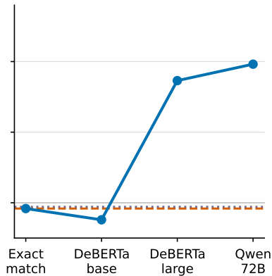
Llama 3.1 70B
