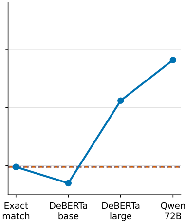
Llama 3.1 8B
