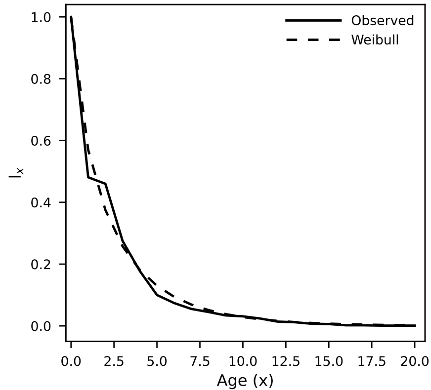
A) Castor canadensis
