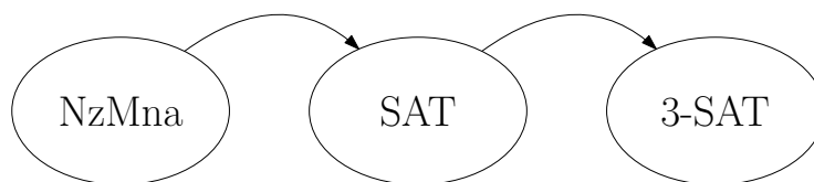
Obrázek 2.4: Idea převodu NzMna \rightarrow 3-SAT.
