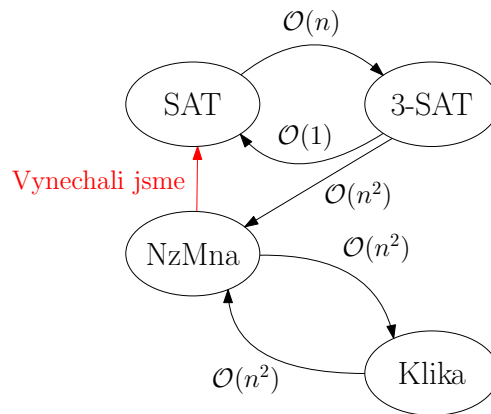
Obrázek 2.10: Shrnutí převodů mezi jednotlivými problémy.
