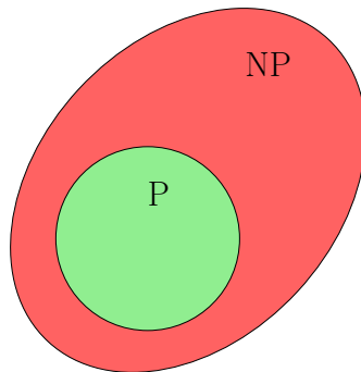
Obrázek 2.11: Ilustrace vztahu P a NP .
