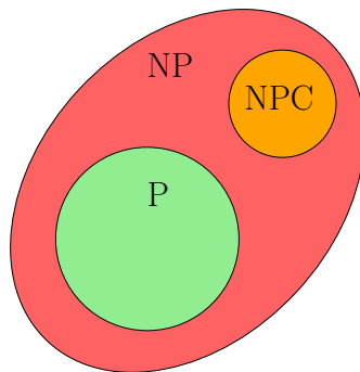
Obrázek 2.12: Ilustrace vztahu P , NP a NPC .
