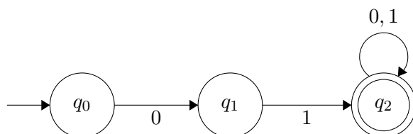
Obrázek 5: Schéma automatu A a tabulka přechodové funkce \delta
