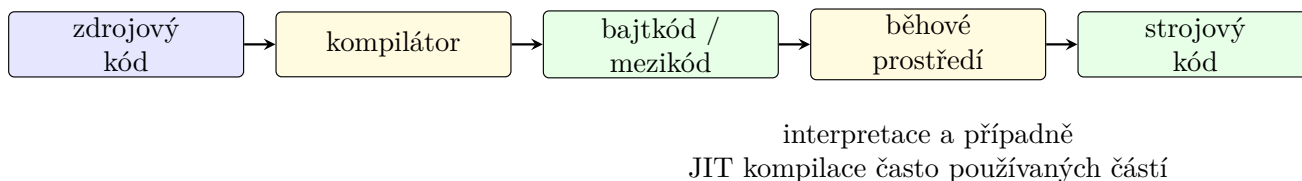
Figure 12: Překlad přes mezikód s možnou JIT kompilací.
