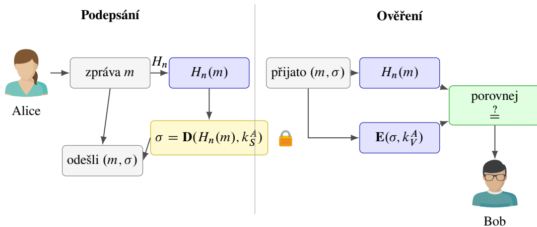
Obrázek 6.21: Podepsání otisku zprávy a následné ověření podpisu.
