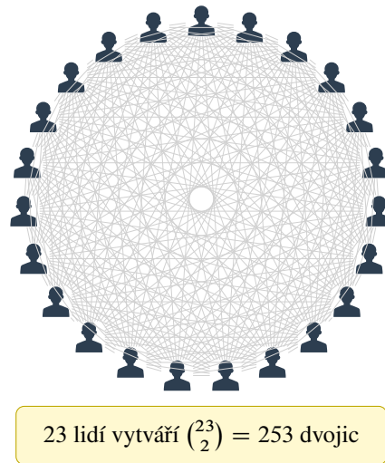
Obrázek 6.16: U 23 lidí porovnááme 253 různých dvojic.
