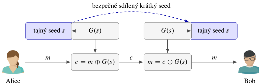
Obrázek 6.14: Použití krátkého seedu k vytvoření dlouhého šifrovacího proudu.
