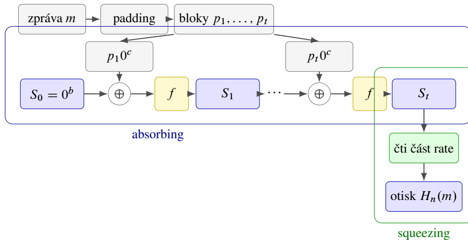
Obrázek 6.19: Fáze absorbing a squeezing konstrukce sponge function.
