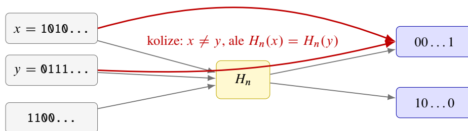
Obrázek 6.15: Více vstupů se musí zobrazit na tentýž n -bitový otisk.
