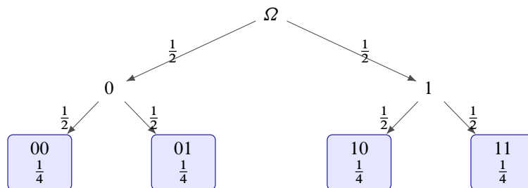
Obrázek 6.3: Dva nezávislé hody mincí a pravděpodobnosti výsledných řetězců.
