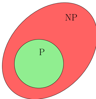
Obrázek 2.12: Ilustrace vztahu P a NP .
