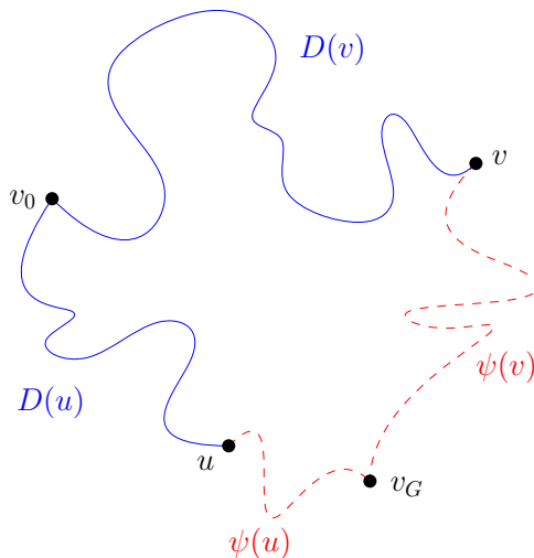
Obrázek 1.19: Znárodnění heuristické funkce \psi .
