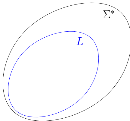
Obrázek 3.4: Obecný jazyk L nad abecedou \Sigma .
