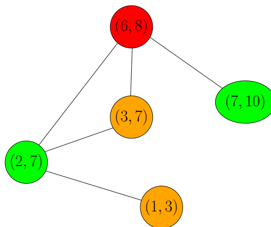
Obrázek 2.6: Obarvení intervalového grafu pro intervaly (2, 7) , (6, 8) , (7, 10) , (1, 3) , (3, 7) .
