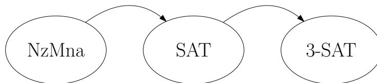
Obrázek 2.4: Idea převodu \text{NzMna} \rightarrow 3\text{-SAT} .
