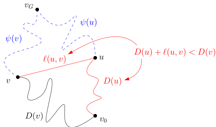
Obrázek 1.20: Situace při výběru vrcholu v při heuristice \psi , kdy D(v) neodpovídá délce nejkratší cesty.
