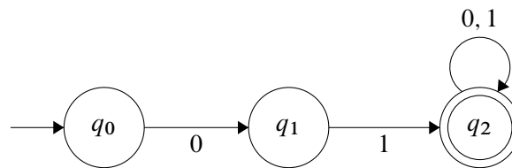
Obrázek 3.5: Schéma automatu A a tabulka přejímové funkce \delta
