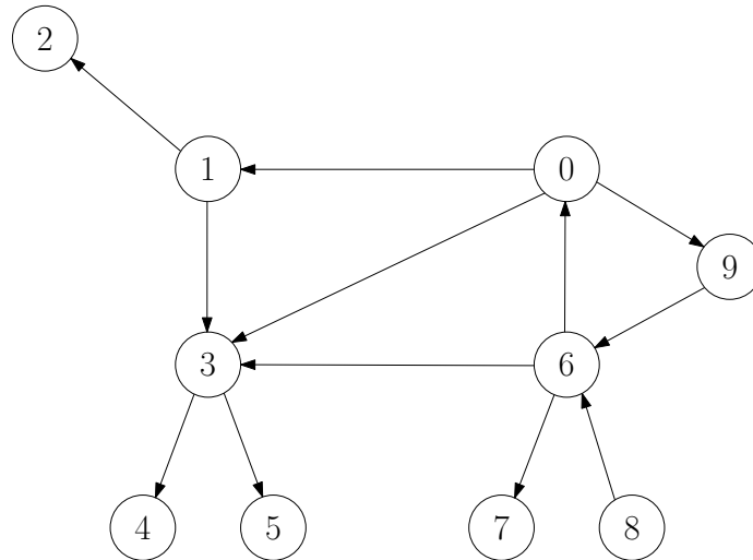
Obrázek 1.2: Prasátkový graf.
