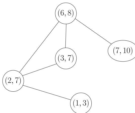
Obrázek 2.6: Příklad intervalového grafu pro intervaly (2, 7), (6, 8), (7, 10), (1, 3), (3, 7) .
