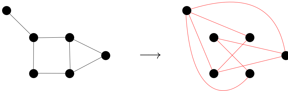
Obrázek 2.10: Doplňek prasátkového grafu.
