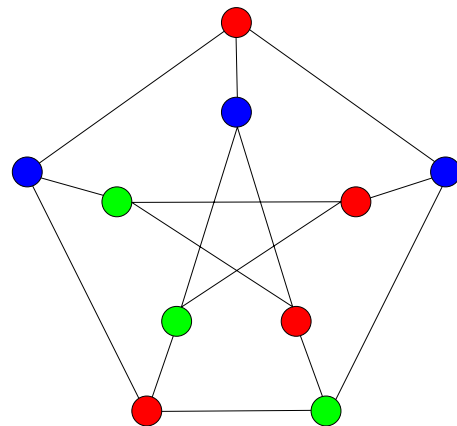
(b) Barvení grafu pro k = 3 .
