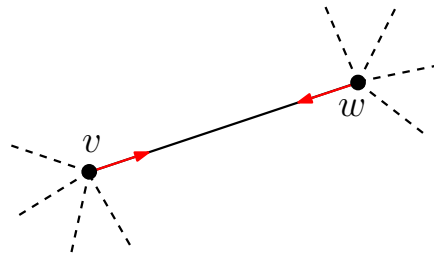
Obrázek 9: Znázornění situace v důkazu části ?? věty ??.
