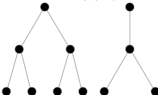
(c) Příklad nekorektního stromu (porušena souvislost).
