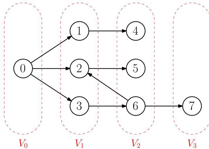
Obrázek 8: Vrcholy rozdělené do vrstev podle průběhu BFS.
