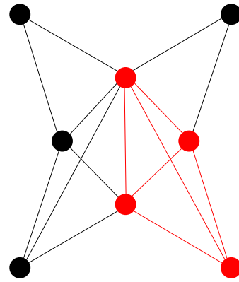
(b) Klika v grafu G_2 .
