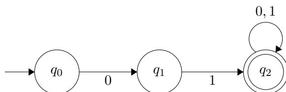
Obrázek 3.5: Schéma automatu A a tabulka přechodové funkce \delta
