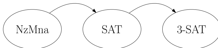
Obrázek 2.5: Idea převodu \text{NzMna} \rightarrow 3\text{-SAT} .
