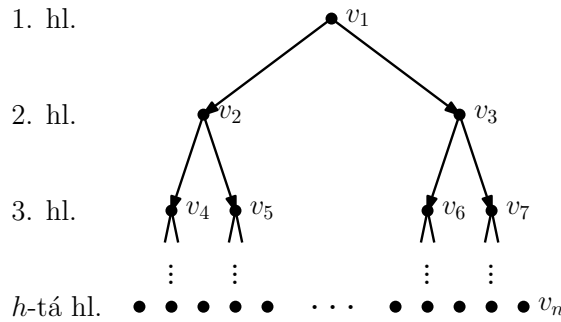
Obrázek 13: Plná binární halda s obecně h hladinami.
