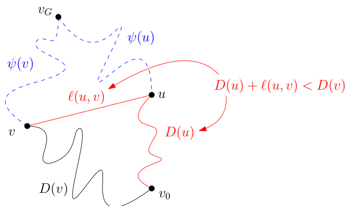
Obrázek 20: Situace při výběru vrcholu v při heuristice \psi , kdy D(v) neodpovídá délce nejkratší cesty.
