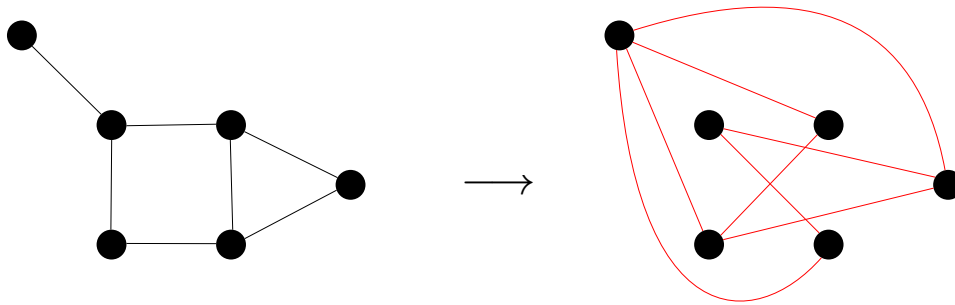
Obrázek 2.10: Doplněk prasátkového grafu.
