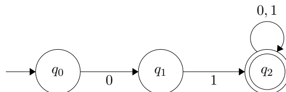
Obrázek 3.5: Schéma automatu A a tabulka přechodové funkce \delta
