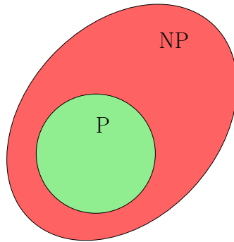
Obrázek 2.12: Ilustrace vztahu P a NP .
