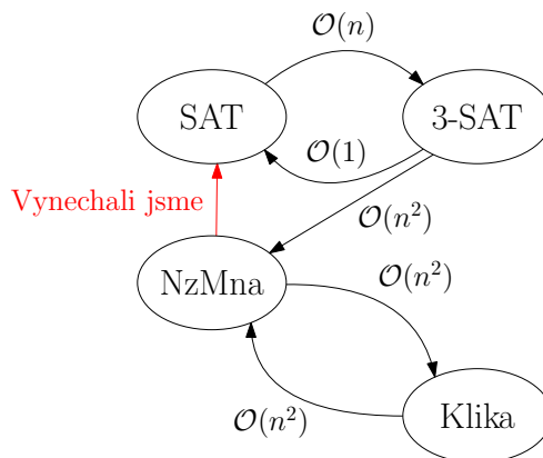
Obrázek 2.11: Shrnutí převodů mezi jednotlivými problémy.
