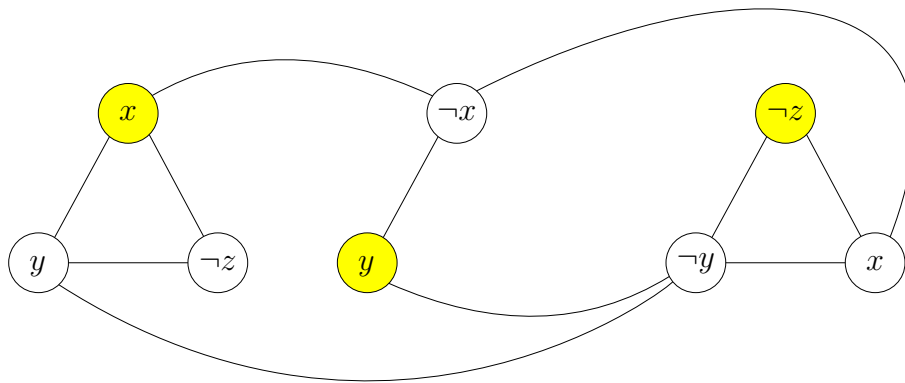
Obrázek 2.4: Ukázka nezávislé množiny příslušné splňujícím literálům pro formuli \psi .
