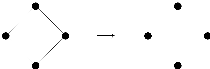
Obrázek 2.9: Doplňek grafu na čtyřech vrcholech.
