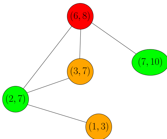
Obrázek 2.7: Obarvení intervalového grafu pro intervaly (2, 7) , (6, 8) , (7, 10) , (1, 3) , (3, 7) .
