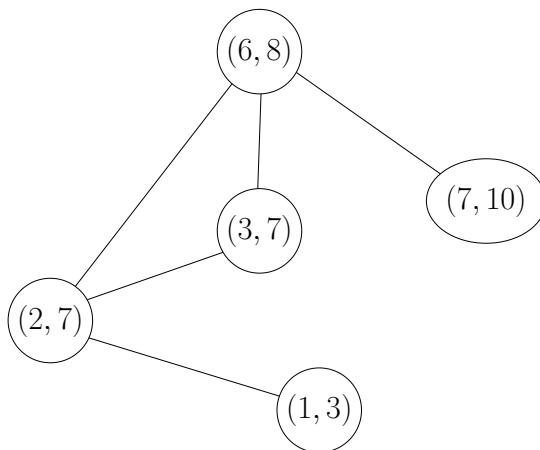
Obrázek 2.6: Příklad intervalového grafu pro intervaly (2, 7) , (6, 8) , (7, 10) , (1, 3) , (3, 7) .
