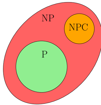
Obrázek 2.13: Ilustrace vztahu P, NP a NPC.
