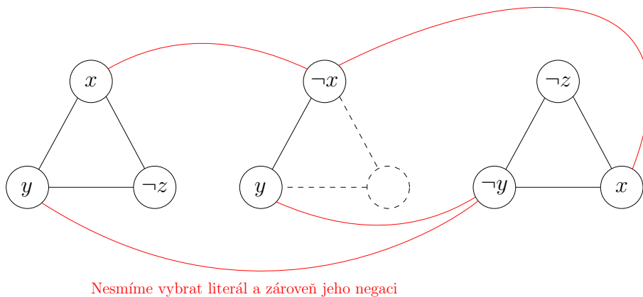
Obrázek 2.3: Ukázka sestaveného grafu pro formuli \psi .
