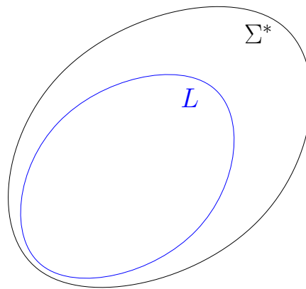
Obrázek 3.4: Obecný jazyk L nad abecedou \Sigma .
