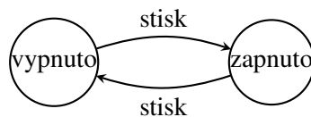
Obrázek 1: Jednoduchý stavový model spínače.
