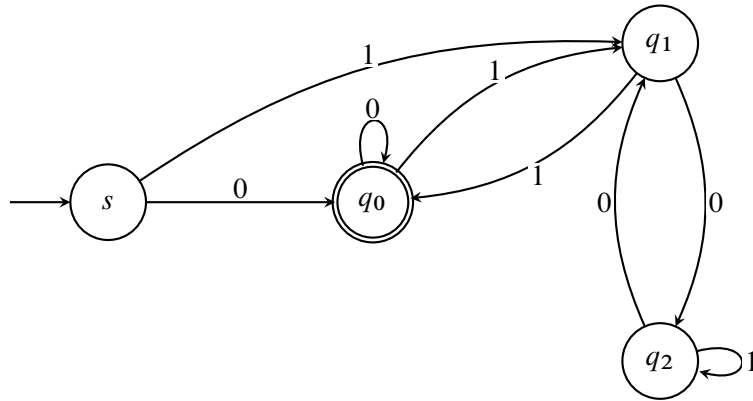
Obrázek 8: DFA pro neprázdné binární zápisy čísel dělitelných třemi.
