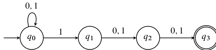
Obrázek 10: NFA pro jazyk slov, jejichž třetí znak od konce je 1.
