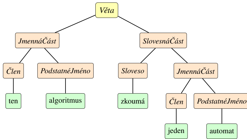
Obrázek 18: Derivační strom věty „ten algoritmus zkoumá jeden automat“.
