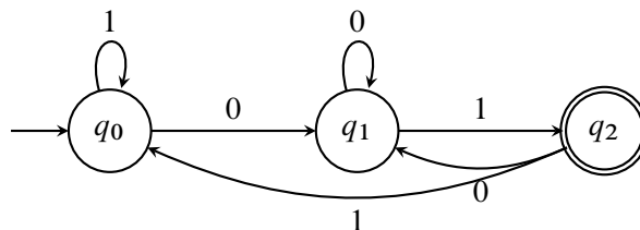
Obrázek 6: DFA pro jazyk L_{\text{suff}} = \{u01 : u \in \{0, 1\}^*\} .
