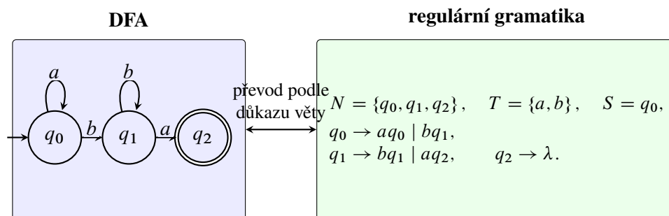
Obrázek 19: Ukázka převodu DFA na ekvivalentní regulární gramatiku.
