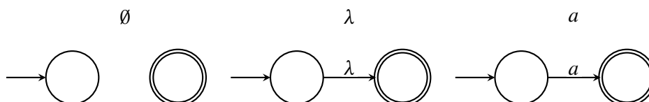
Obrázek 13: Základní automaty pro výrazy \emptyset , \lambda a a .
