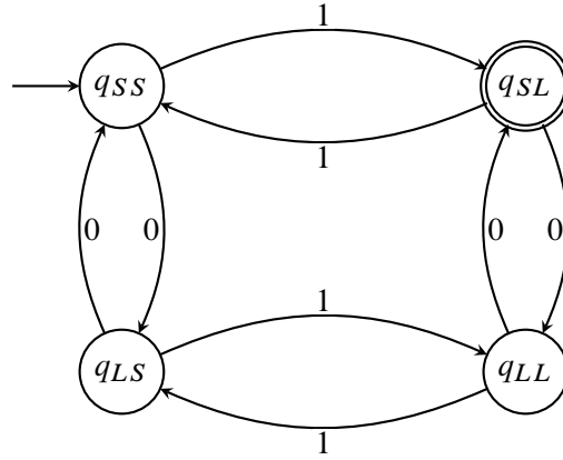
Obrázek 7: DFA přijímající slova se sudým počtem nul a lichým počtem jedniček.
