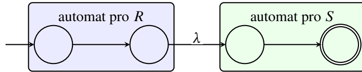
Obrázek 15: Konstrukce automatu pro zřetězení RS .
