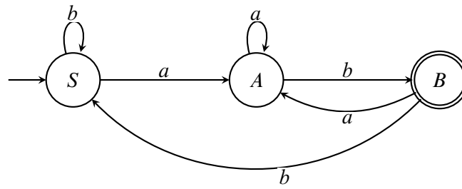
Obrázek 20: DFA pro slova končící na ab .
