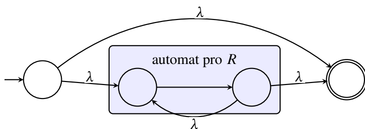
Obrázek 16: Konstrukce automatu pro Kleeneho hvězdu R^* .
