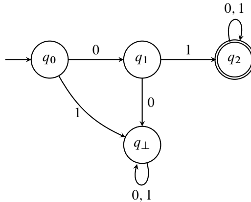
Obrázek 5: DFA přijímající právě slova začínající na 01.
