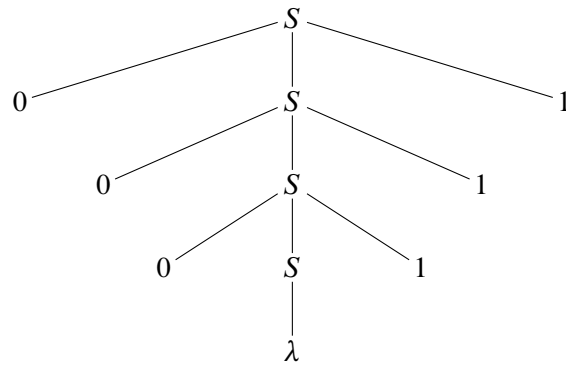
Obrázek 17: Derivační strom pro slovo 000111 v gramatice S \rightarrow 0S1 \mid \lambda .
