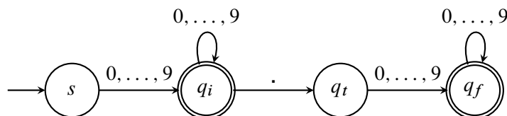
Obrázek 11: Konečný automat pro jednoduchý zápis nezáporného desetinného čísla.
