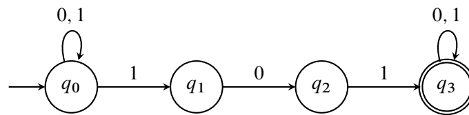
Obrázek 9: NFA přijímající právě slova obsahující podslovo 101.
