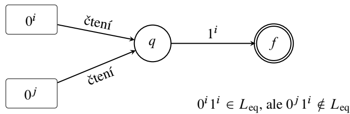
Obrázek 12: Po slovech 0^i a 0^j je automat ve stejném stavu, takže stejný konec 1^i už nedokáže rozlišit.
