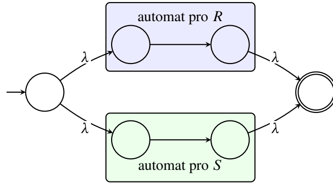
Obrázek 14: Konstrukce automatu pro sjednocení R \mid S .
