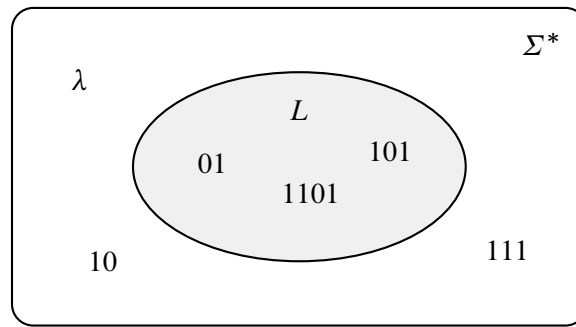
Obrázek 4: Jazyk L je libovolná podmnožina množiny všech slov \Sigma^* .
