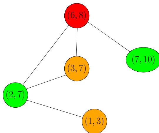
Obrázek 2.6: Obarvení intervalového grafu pro intervaly (2, 7) , (6, 8) , (7, 10) , (1, 3) , (3, 7) .
