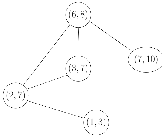
Obrázek 2.5: Příklad intervalového grafu pro intervaly (2, 7) , (6, 8) , (7, 10) , (1, 3) , (3, 7) .
